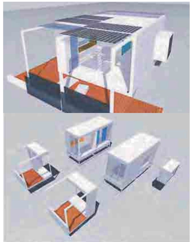
Conjunto de módulos a ensamblar en obra.
